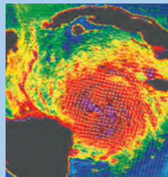
Mesoscale Winds
